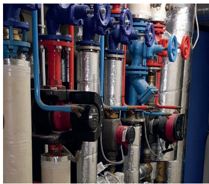
Die neue Heizungsanlage mit Warmwasserbereitung
